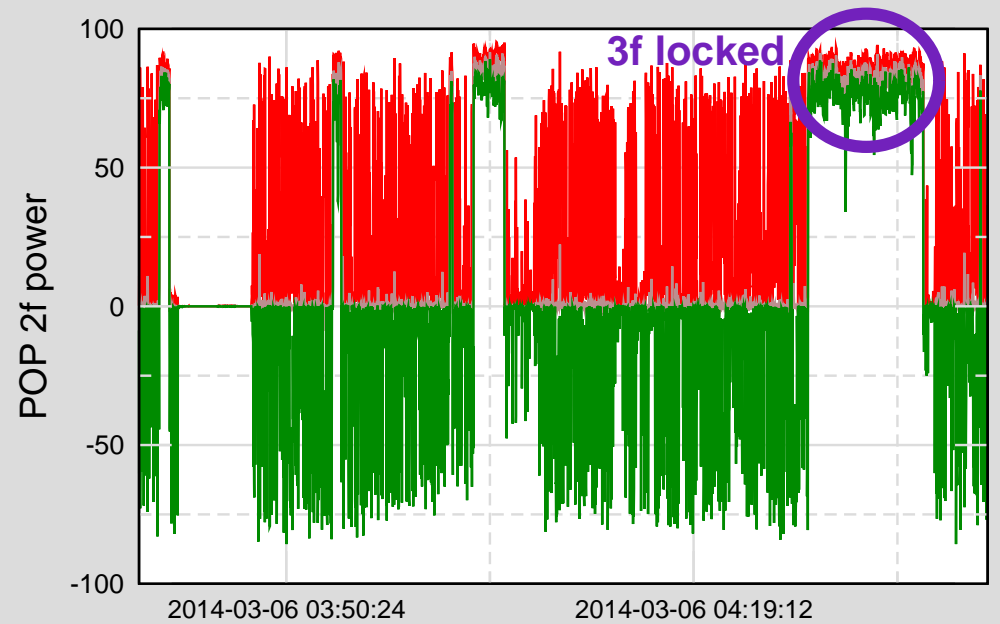
H1:LSC-POPAIR_B_RF18_I_ERR_DQ
