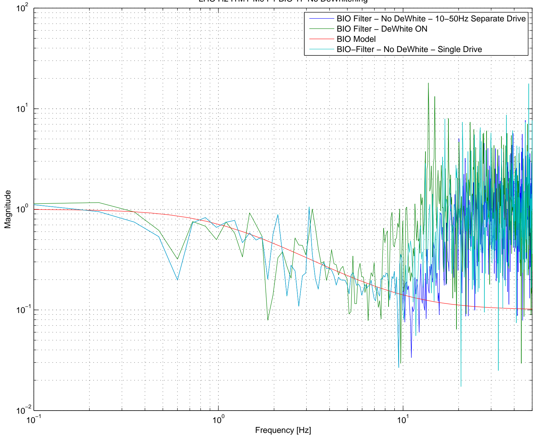
LHO H2 ITMY M0 F1 BIO TF No DeWhitening
