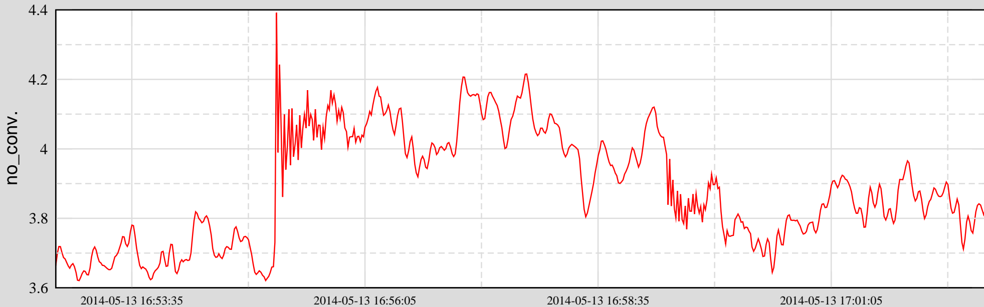
Ch 2: H1:SUS-ETMY_L3_OPLEV_YAW_OUT_DQ
