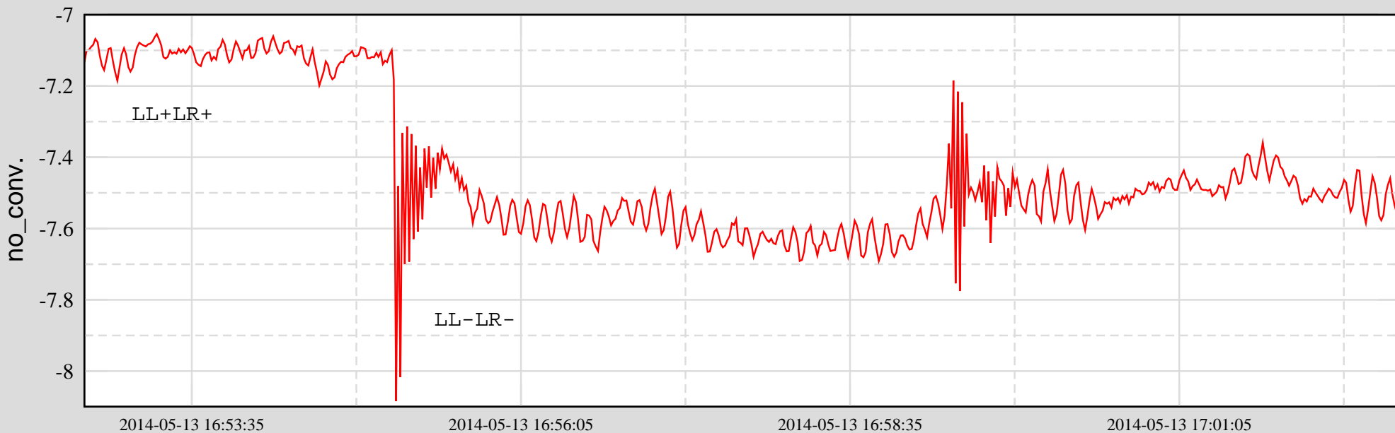
Ch 1: H1:SUS-ETMY_L3_OPLEV_PIT_OUT_DQ
