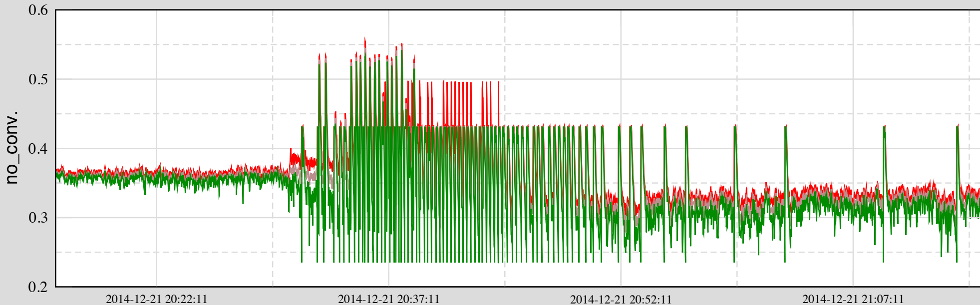
Ch 9: H1:PSL-ISS_AOM_DRIVER_MON_OUT_DQ
