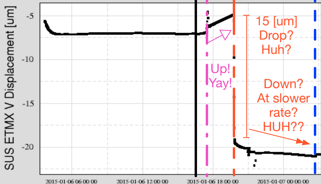
Ch 1: H1:SUS-ETMX_M0_DAMP_V_INI_DQ
