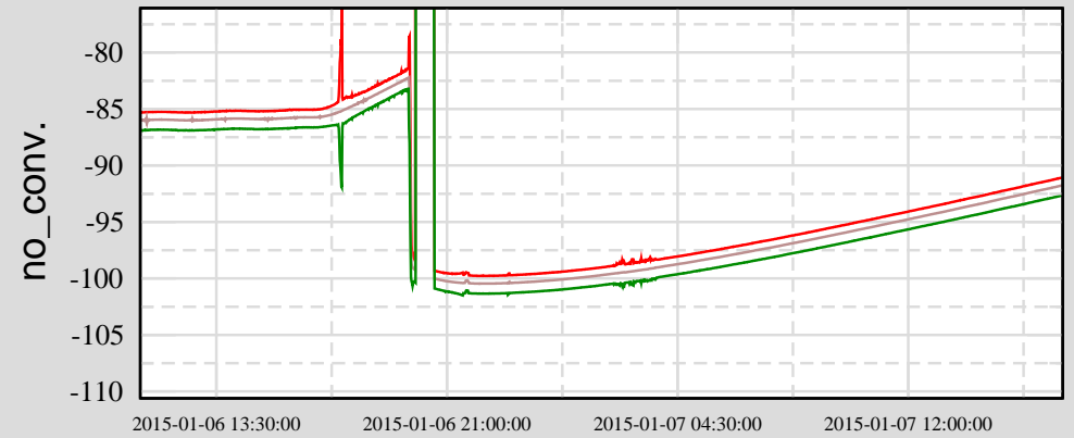
Ch 4: H1:SUS-ETMX_R0_DAMP_V_INMON
