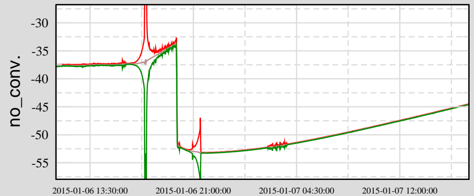
Ch 4: H1:SUS-ETMX_R0_DAMP_V_INMON
