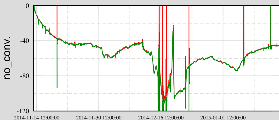
Ch 5: H1:SUS-ETMY_R0_DAMP_V_INMON
