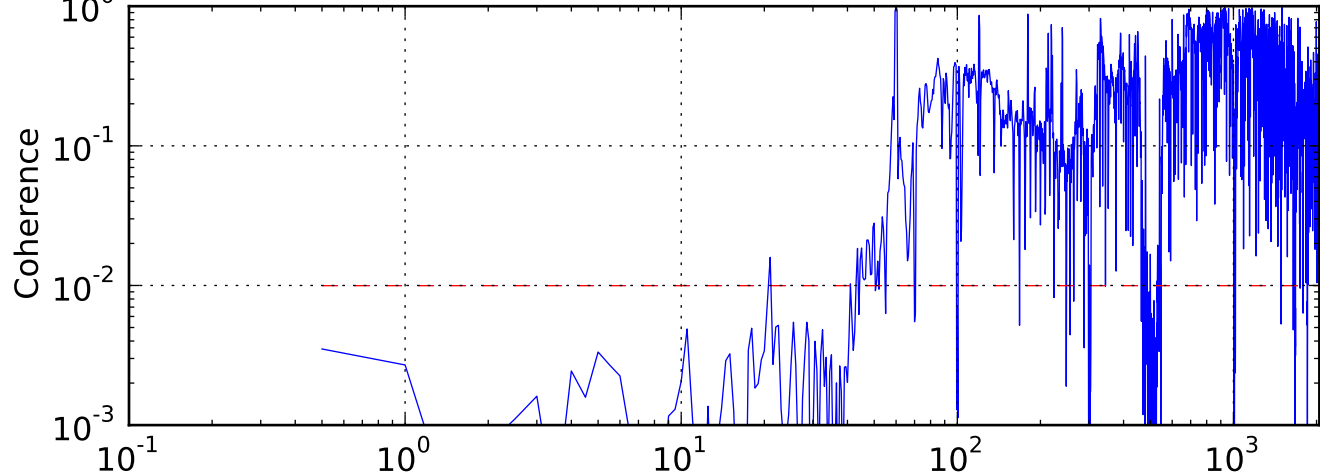
Coherence LSC-DARM_IN1_DQ vs H1:PSL-ISS_SECONDLOOP_SUM14_REL_OUT_DQ - GPS 1107680416
