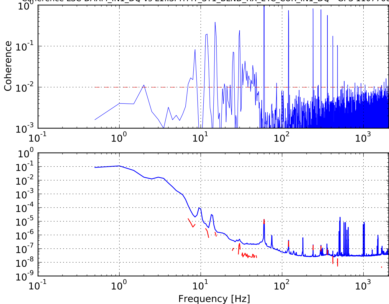
Coherence LSC-DARM_IN1_DQ vs L1:ISI-ITMY_ST1_BLND_RX_L4C_CUR_IN1_DQ - GPS 1107760396
