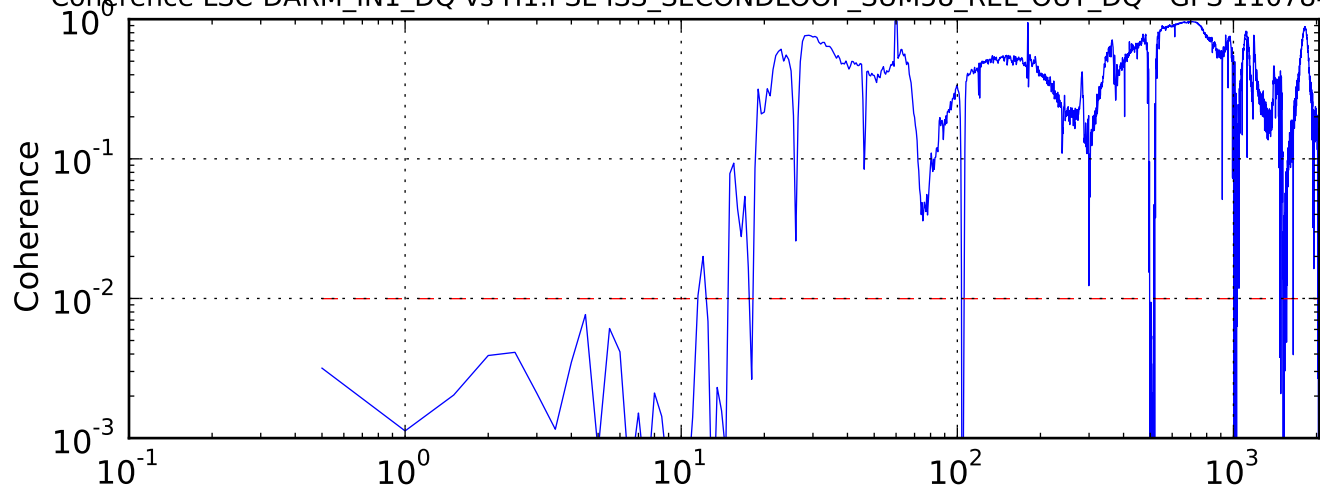
Coherence LSC-DARM_IN1_DQ vs H1:PSL-ISS_SECONDLOOP_SUM58_REL_OUT_DQ - GPS 1107840506
