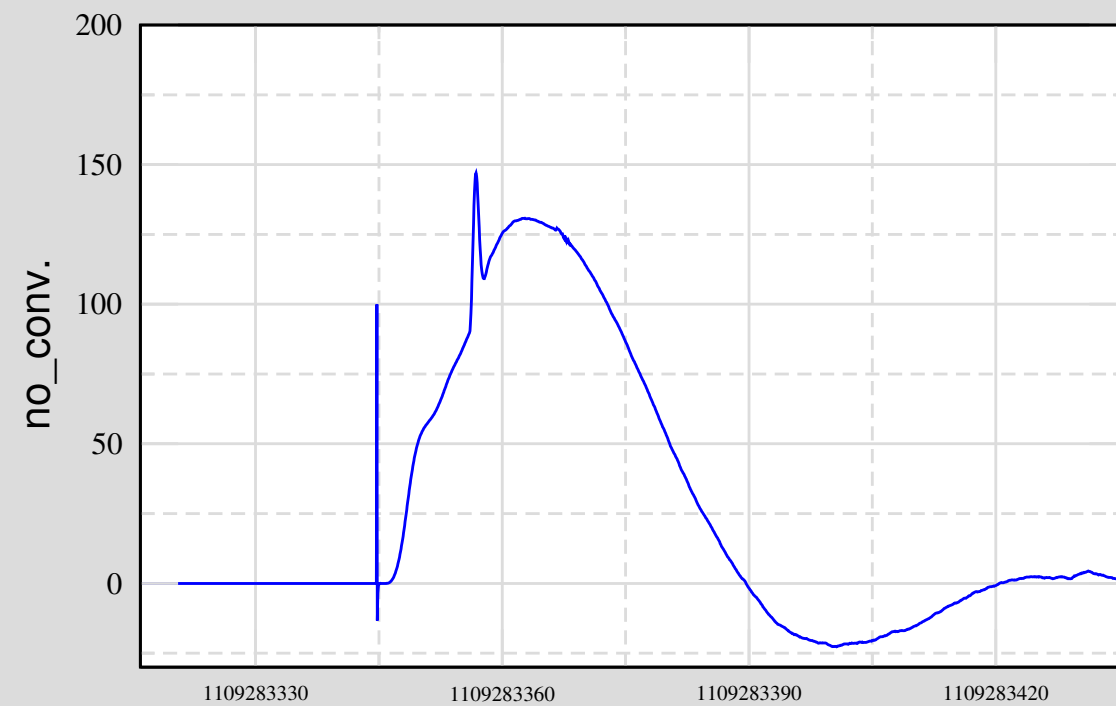
Ch 3: H1:ISI-BS_ST2_ISO_RZ_OUT16
