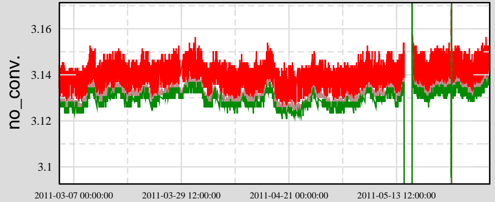
Ch 5: H1:PSL-NPRO_D2PWR
