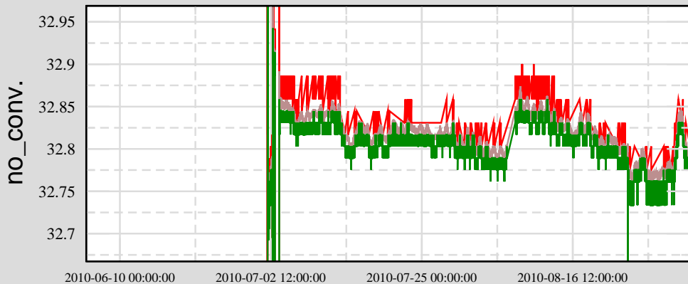
Ch 2: H1:PSL-AMP_D2PWR
