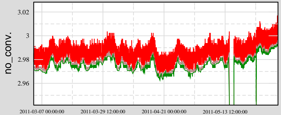
Ch 4: H1:PSL-AMP_D4PWR
