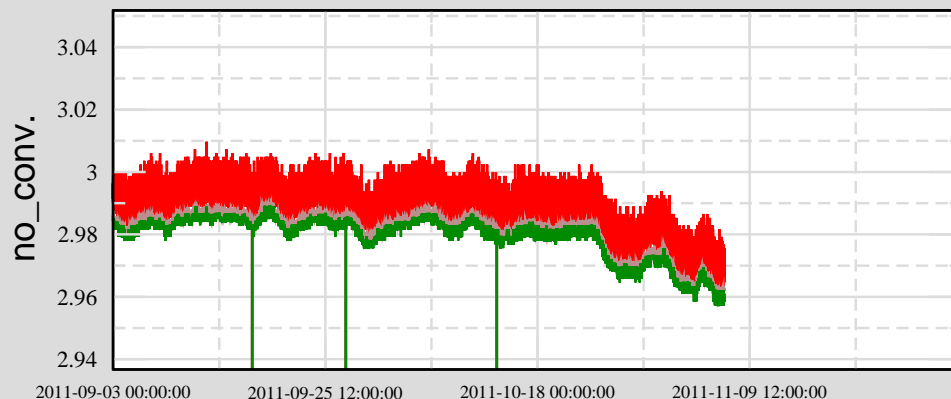
Ch 4: H1:PSL-AMP_D4PWR
