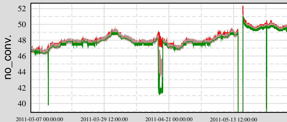
Ch 4: H1:PSL-AMP_PWR2
