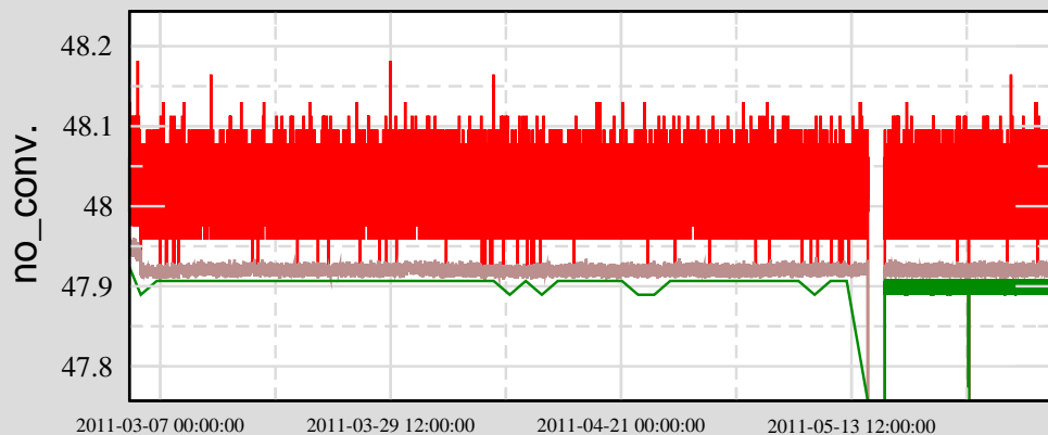
Ch 1: H1:PSL-AMP_DCUR1
