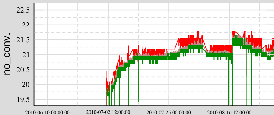
Ch 4: H1:PSL-AMP_PWR2
