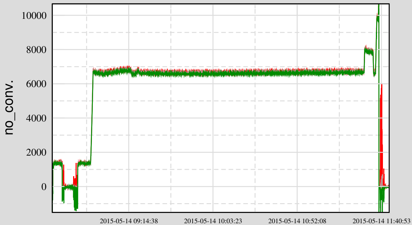
Ch 2: H1:LSC-ASAIR_B_RF90_I_ERR_DQ
