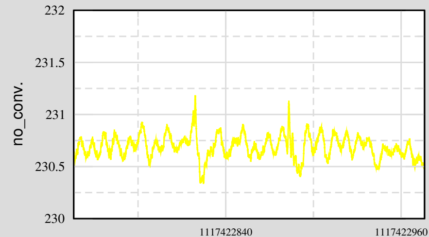
Ch 4: H1:SUS-MC2_M2_WIT_P_DQ
