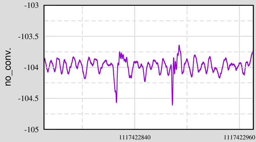
Ch 5: H1:SUS-MC2_M2_WIT_Y_DQ
