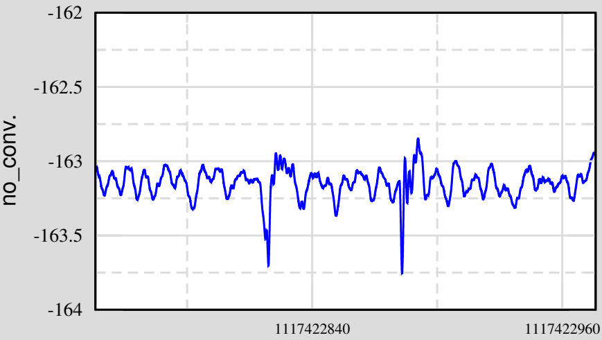
Ch 2: H1:SUS-MC2_M3_WIT_Y_DQ
