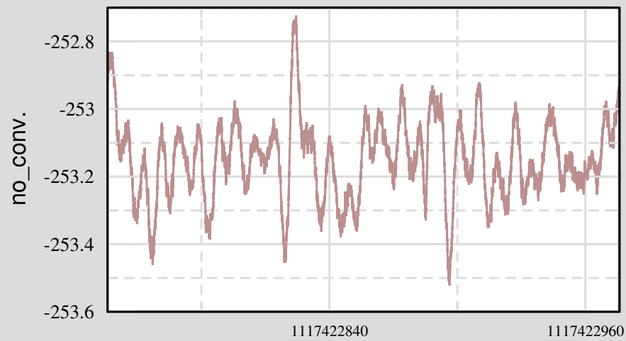
Ch 4: H1:SUS-MC2_M2_WIT_P_DQ
