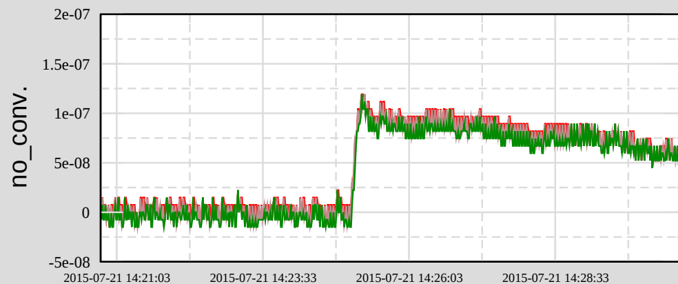
Ch 4: H1:SYS-TIMING_C_MA_A_GPSDELAY
