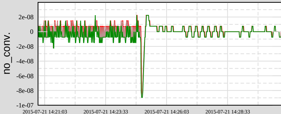
Ch 2: H1:SYS-TIMING_C_MA_A_USEEXT
