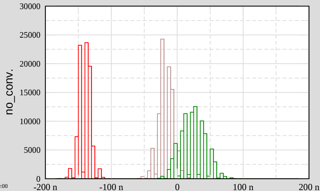
Ch 10: H1:SYS-TIMING_C_MA_A_PORT_2_SLAVE_CFC_TIMEDIFF_4
