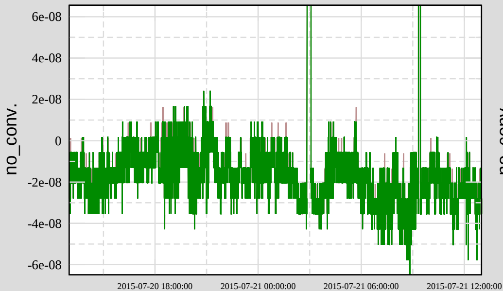
Ch 8: H1:SYS-TIMING_C_MA_A_PORT_2_SLAVE_CFC_TIMEDIFF_2
