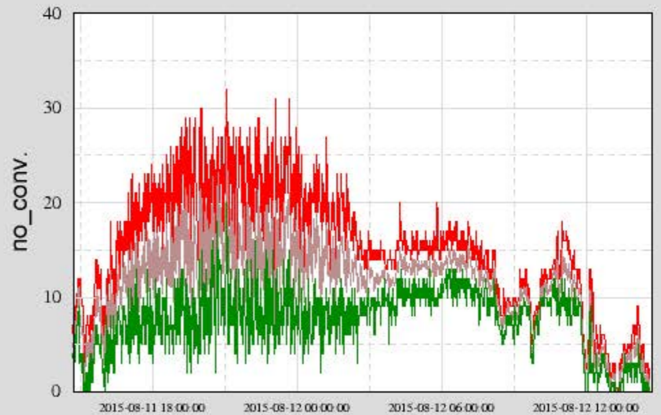
Ch 3: H1:PEM-EY_WIND_ROOF_WEATHER_MPH
