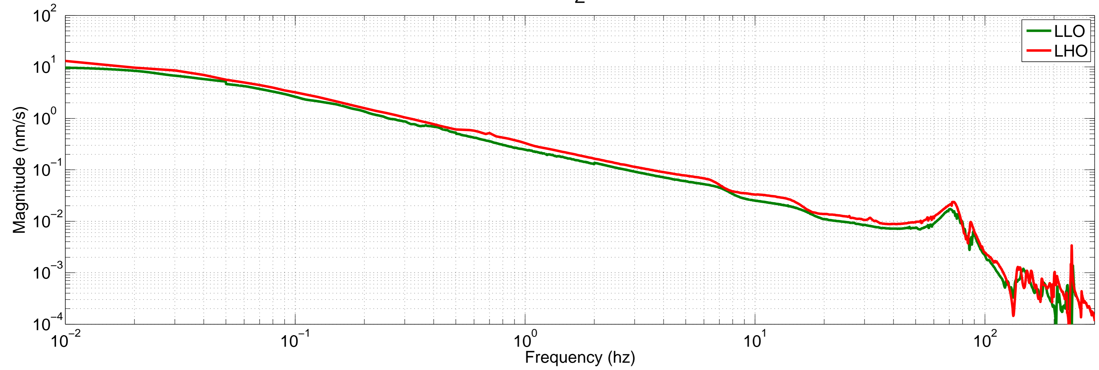
LLO & LHO HAM1 HEPI Cart TFs Z
