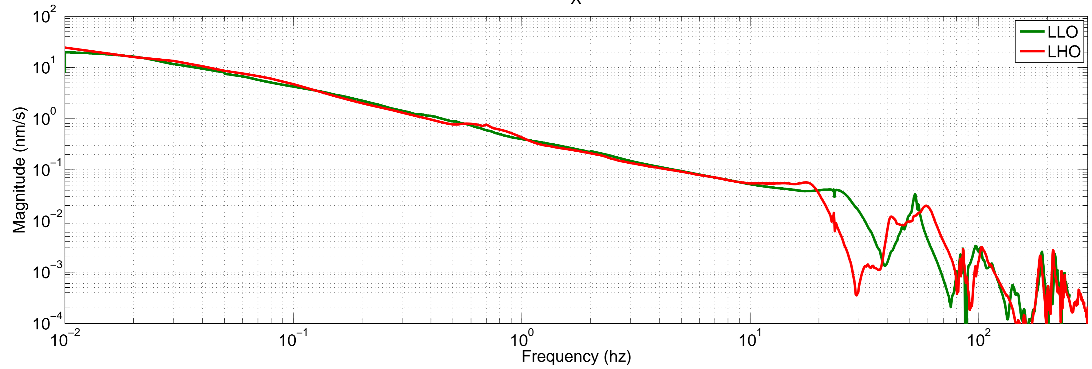
LLO & LHO HAM1 HEPI Cart TFs X
