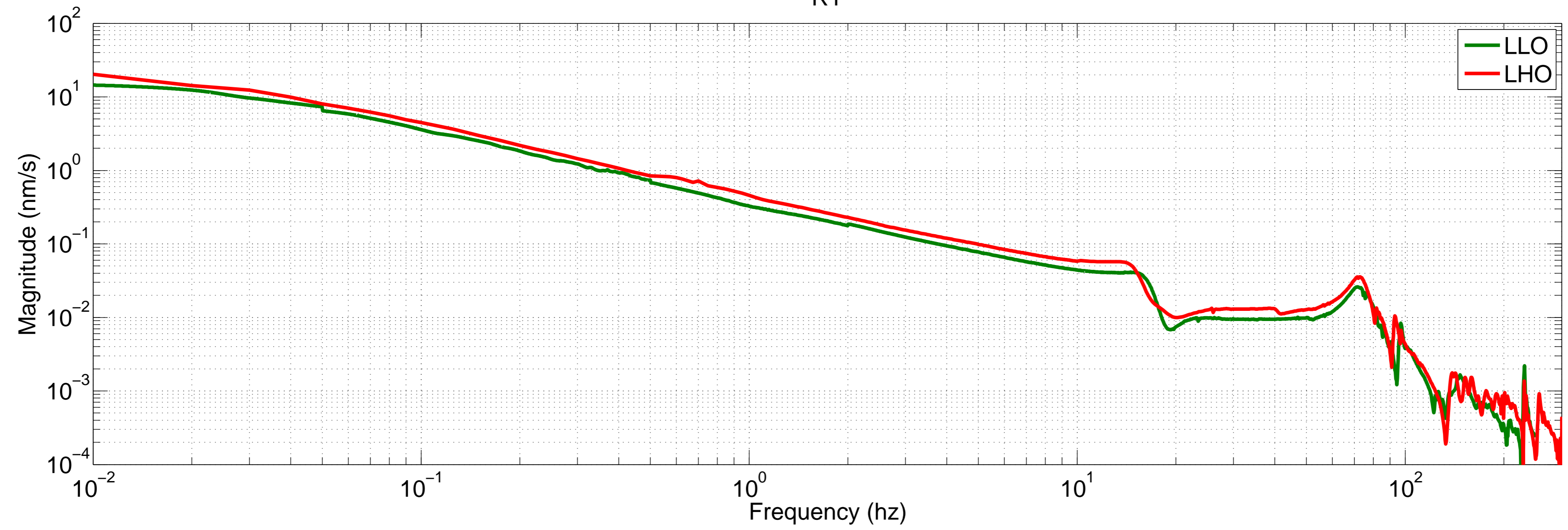
LLO & LHO HAM1 HEPI Cart TFs RY
