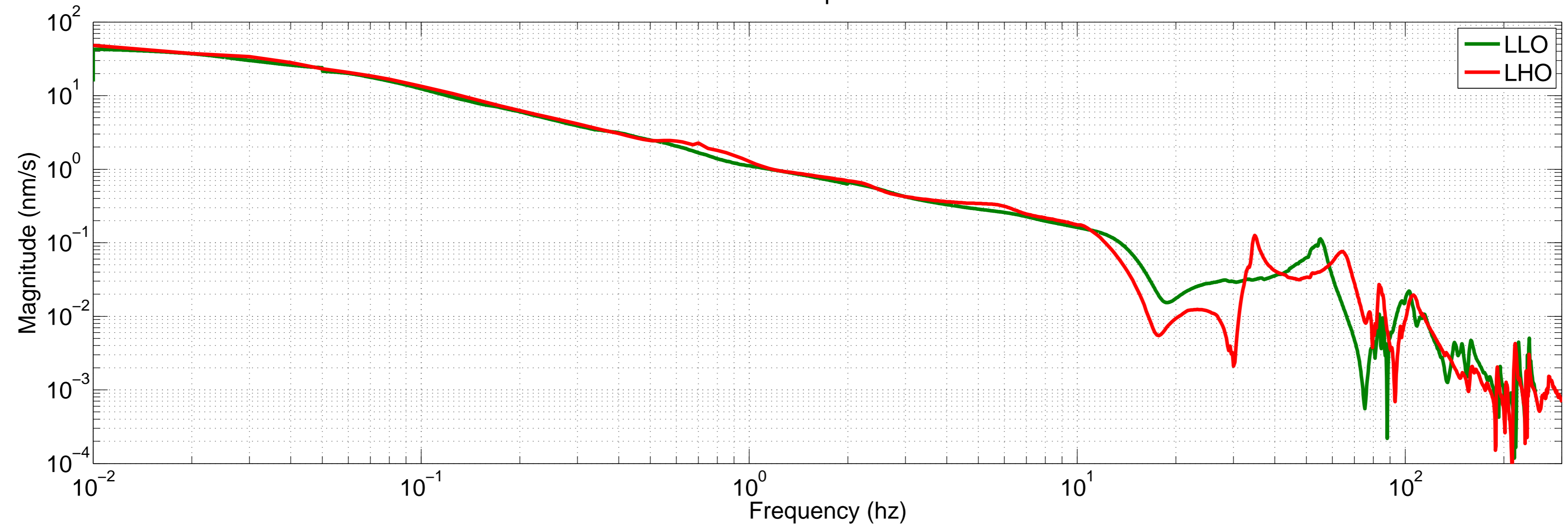
LLO & LHO HAM1 HEPI Cart TFs Y
