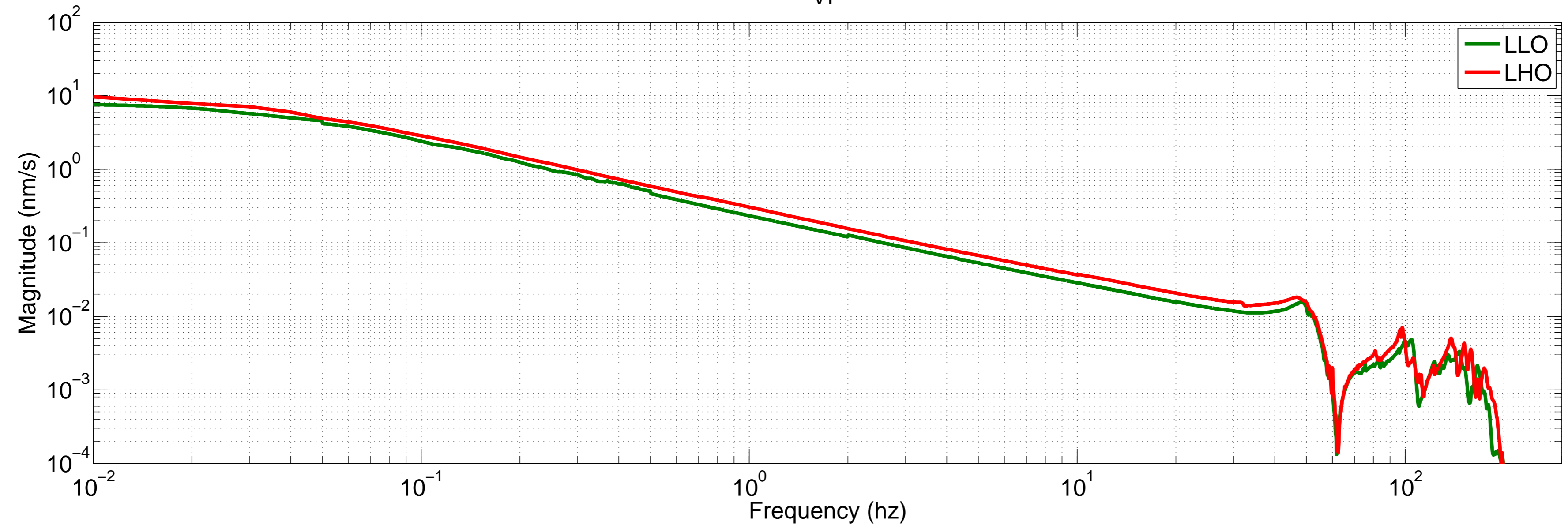
LLO & LHO HAM1 HEPI Cart TFs VP
