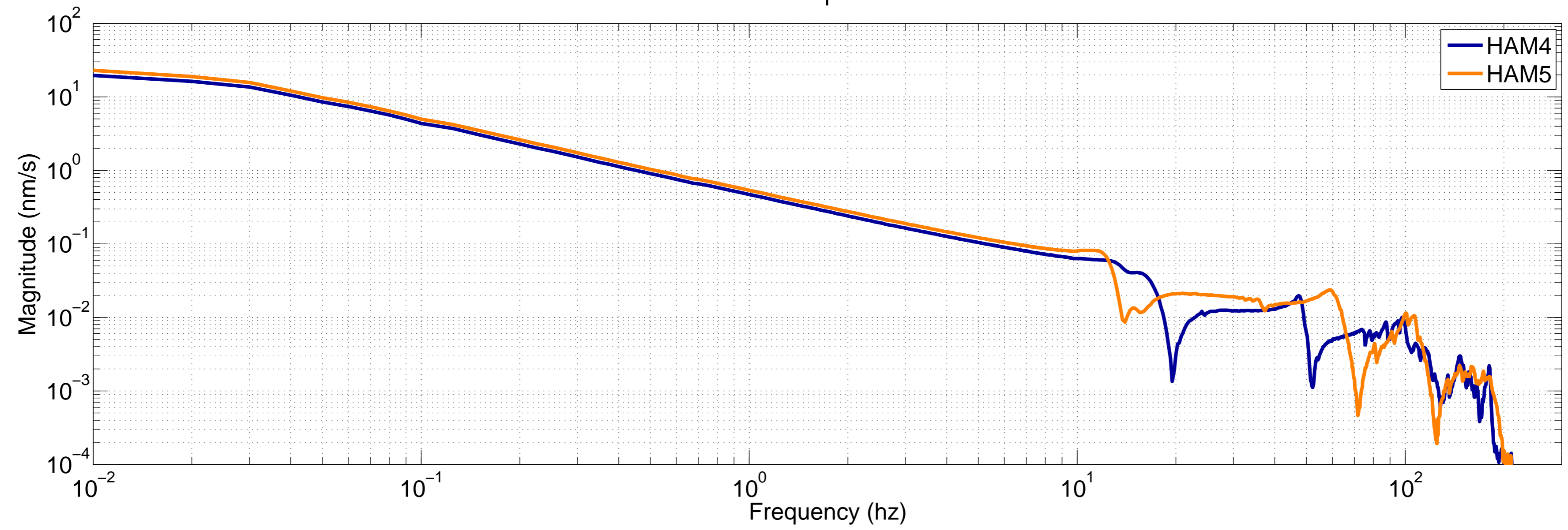
LHO HAM4 & HAM5 HEPI Cart TFs Y
