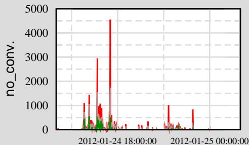
Ch 11: H0:PEM-EY_DST2_5
