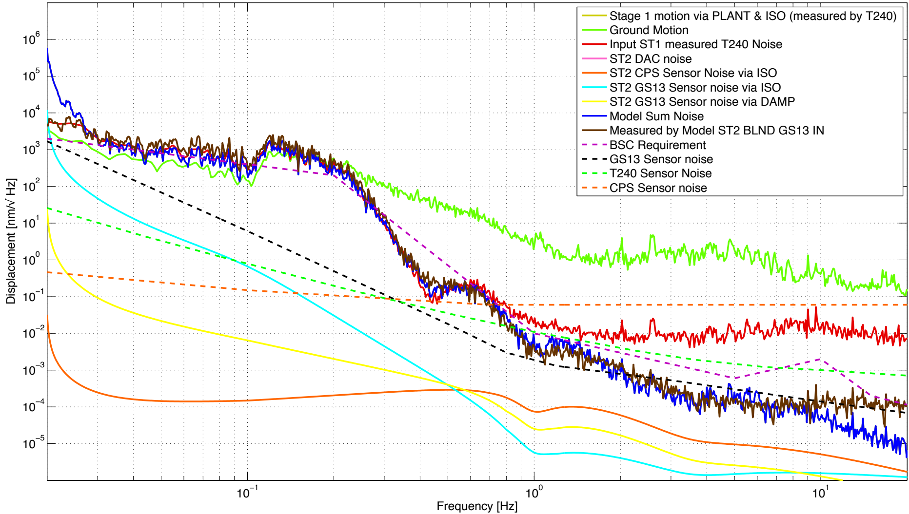
ITMY -ST2 GS13 Y IN1 for GPS 1125042762
