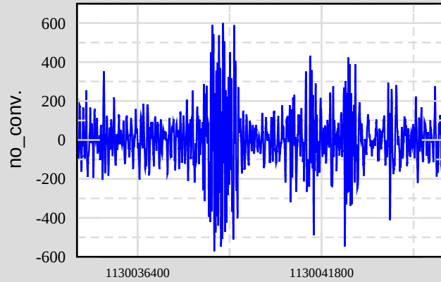
Ch 2: H1:ASC-CHARD_Y_OUT_DQ
