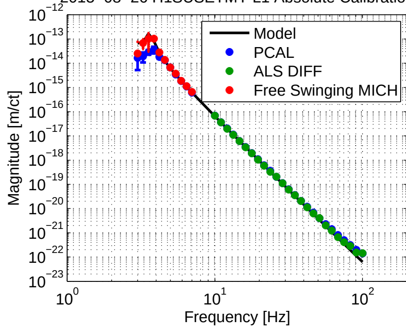
2015-08-26 H1SUSETMY L1 Absolute Calibration
