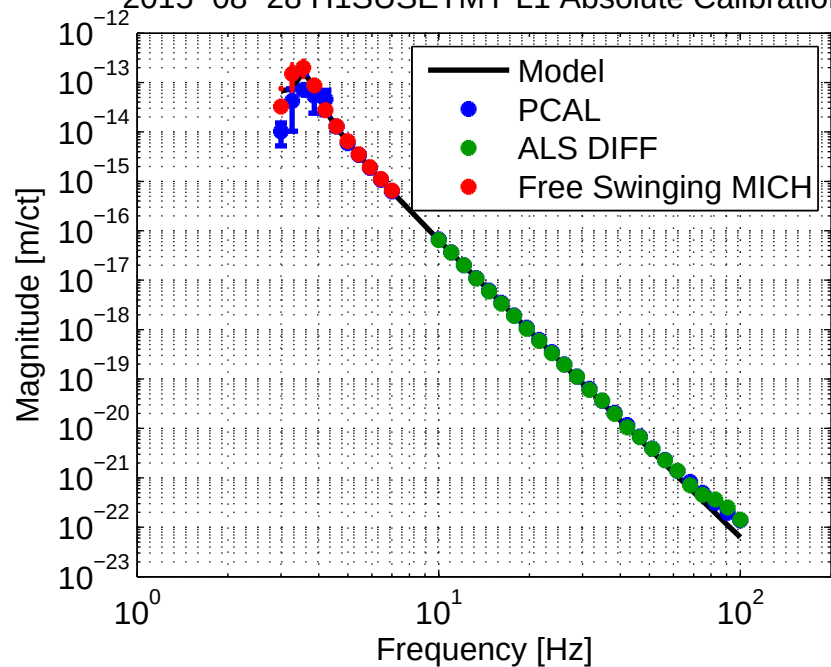
2015-08-28 H1SUSETMY L1 Absolute Calibration
