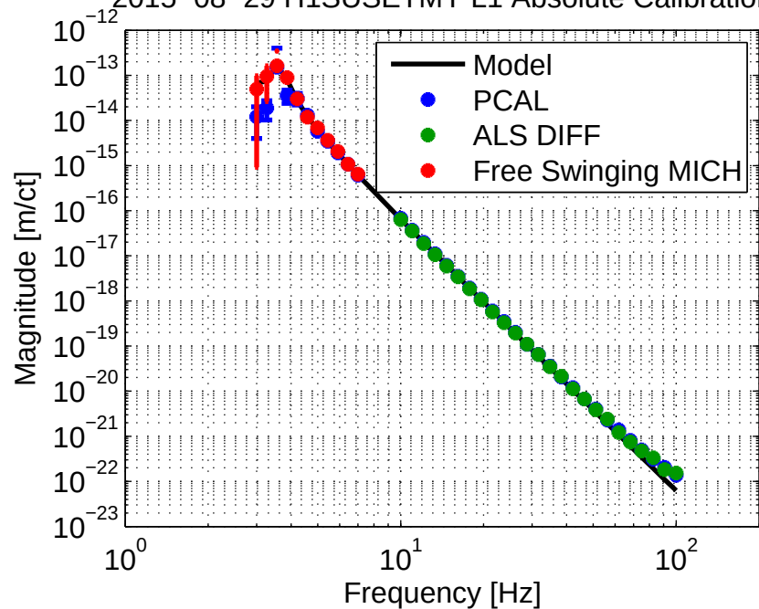
2015-08-29 H1SUSETMY L1 Absolute Calibration
