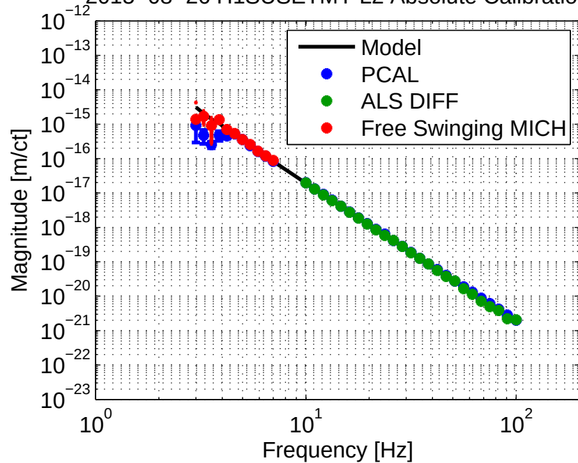
2015-08-26 H1SUSETMY L2 Absolute Calibration
