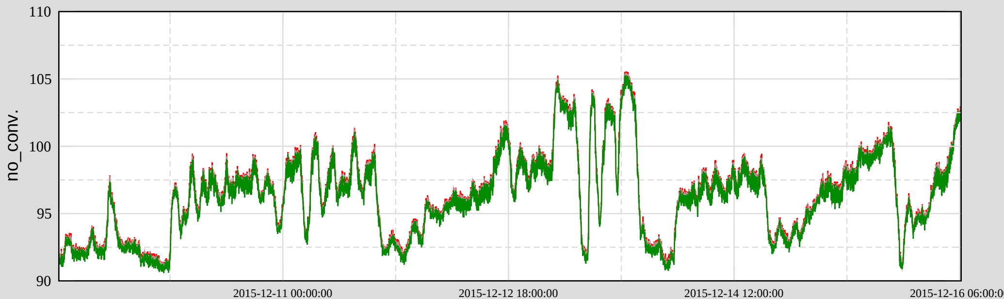
Ch 14: H0:FMC-CS_LVEA_REHEAT_4_DEGF
