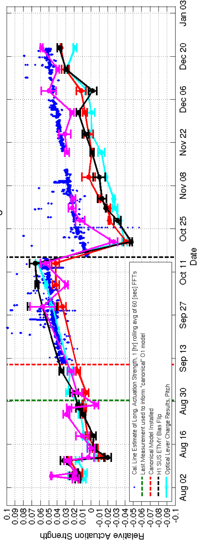
H1 SUS ETMY ESD Actuation Strength Metrics vs. Time
