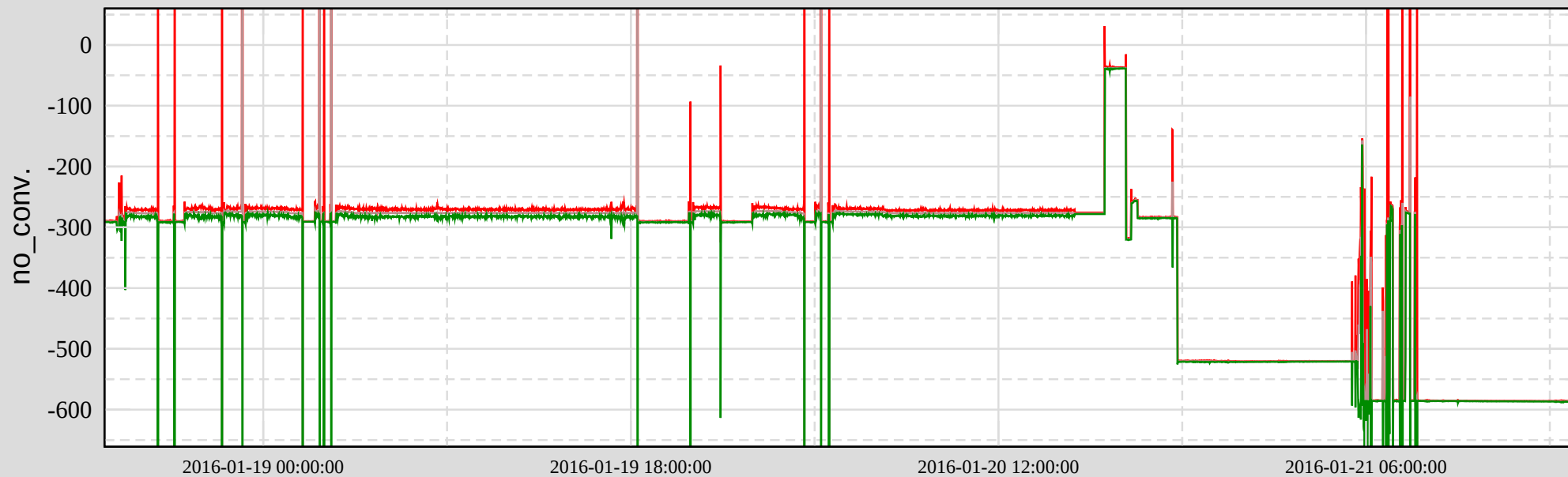
Ch 10: H1:SUS-RM1_M1_DAMP_Y_INMON
