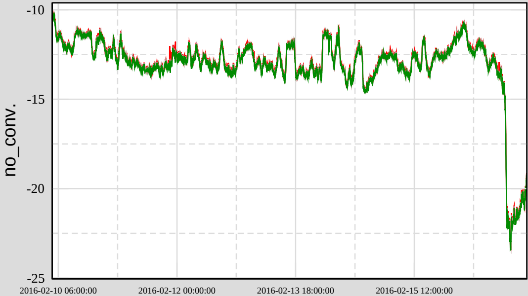
Ch 2: H1:ISI-HAM2_OPLEV_YAW_OUT16
