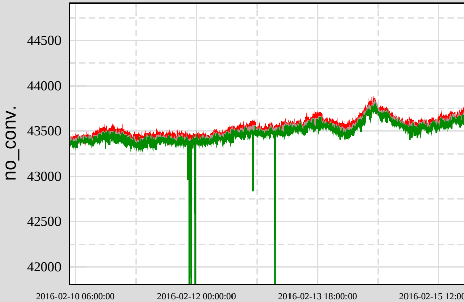
Ch 3: H1:ISI-HAM2_OPLEV_SUM_OUT16
