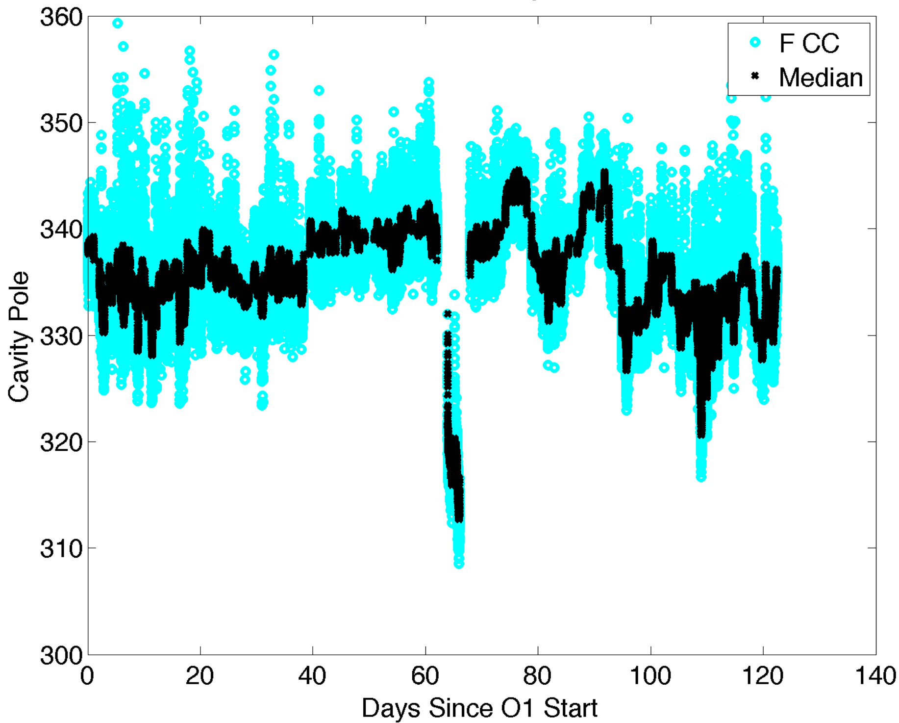
LHO C02 Cavity Pole
