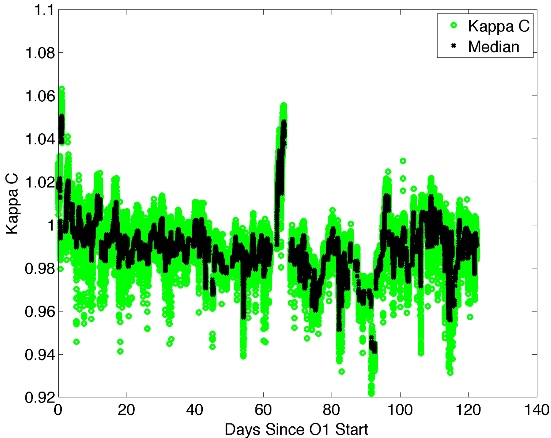
LHO C02 Kappa C
