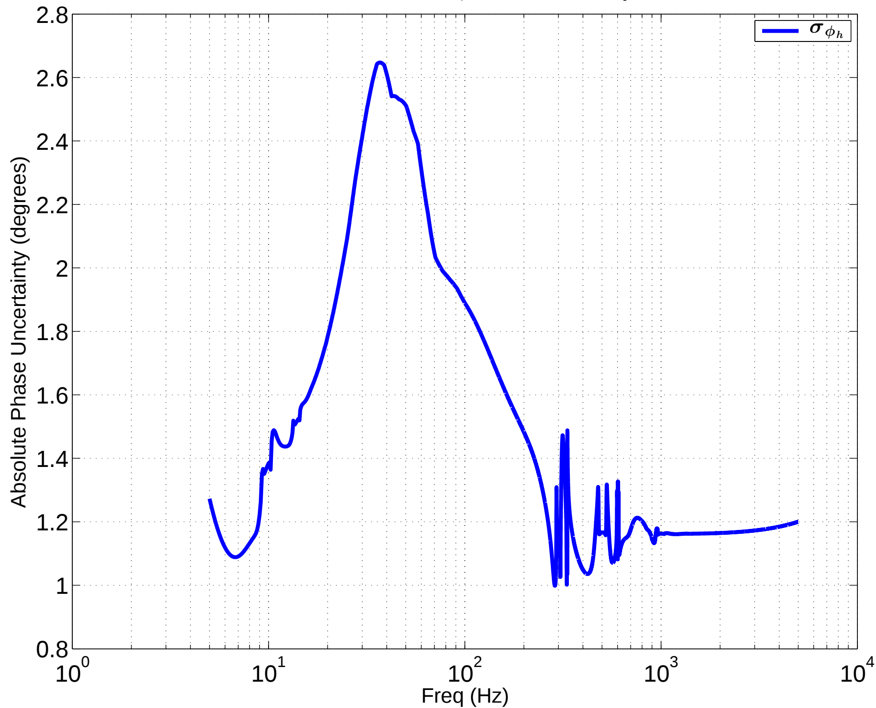
LHO C02 \phi_h Uncertainty
