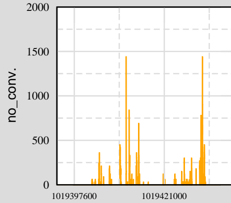
Ch 11: H0:PEM-EY_DST2_5
