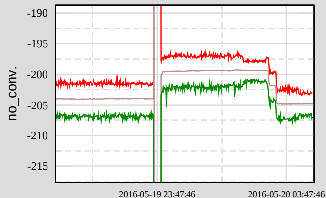
Ch 5: H1:SUS-IM2_M1_DAMP_Y_INMON
