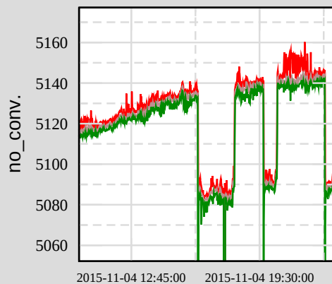
Ch 4: H1:SUS-ITMY_L3_OPLEV_SUM_OUT_DQ
