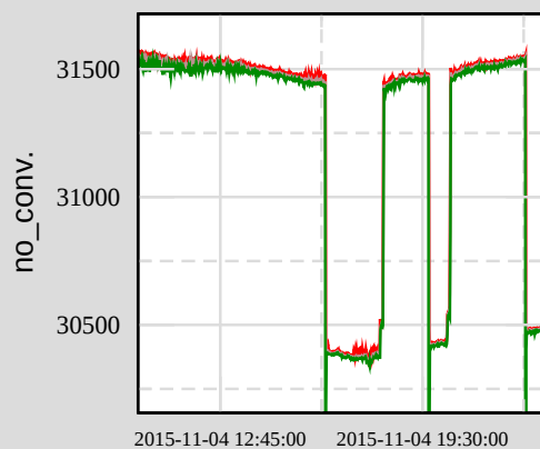
Ch 1: H1:SUS-ETMX_L3_OPLEV_SUM_OUT_DQ
