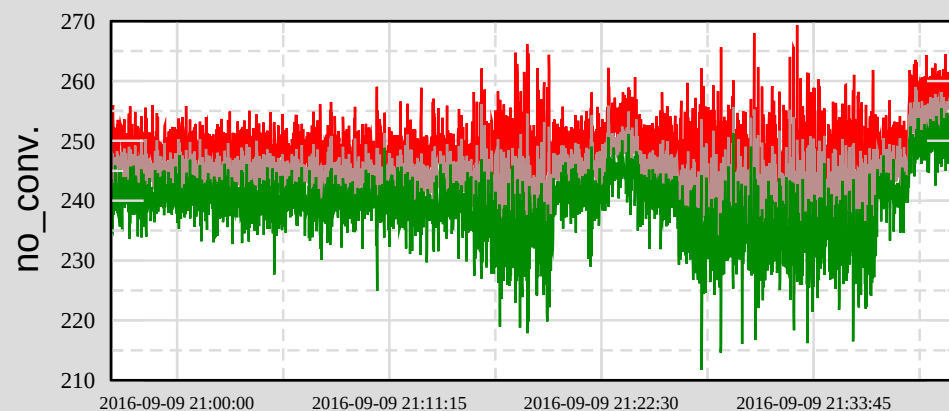
Ch 12: H1:PSL-ISS_OUTERLOOP_OUTPUT_MON
