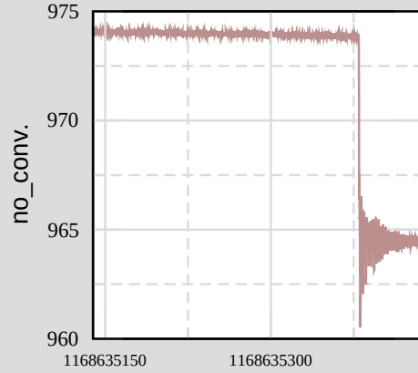
Ch 4: H1:SUS-ITMY_M0_DAMP_R_INMON
