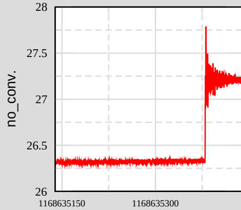
Ch 1: H1:SUS-ITMY_M0_DAMP_L_INMON
