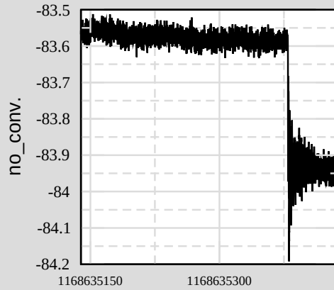
Ch 4: H1:SUS-ITMY_M0_DAMP_R_INMON
