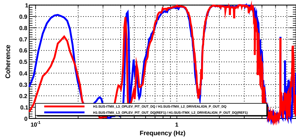
Coherence
