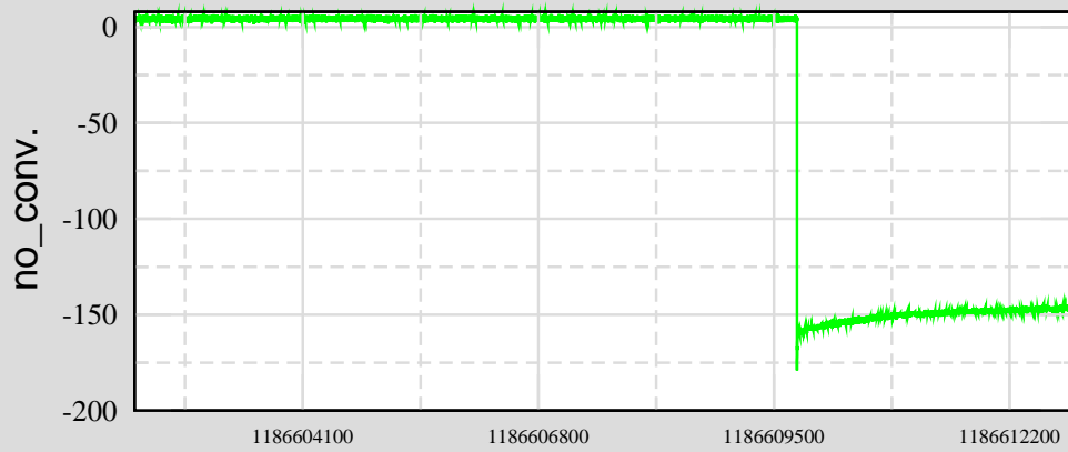
Ch 1: H1:SUS-ETMX_L2_RMSIMON_LL_MON
