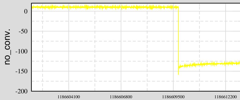
Ch 4: H1:SUS-ETMX_L2_RMSIMON_UR_MON
