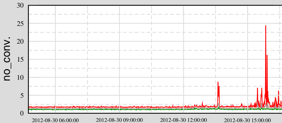
Ch 5: H2:PEM-CS_SEIS_LVEA_FLOOR_X_BLRMS_10HZ30
