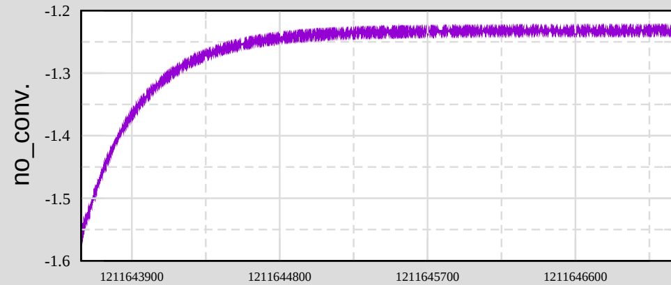
Ch 5: H1:SQZ-OPO_TEC_CURRENTBACK
