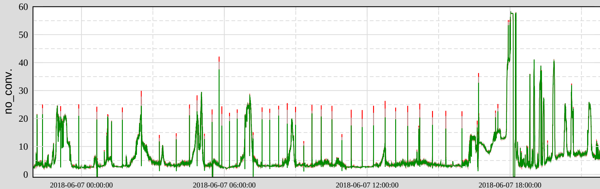
Ch 3: H1:PSL-FSS_PC_MON_OUTPUT
