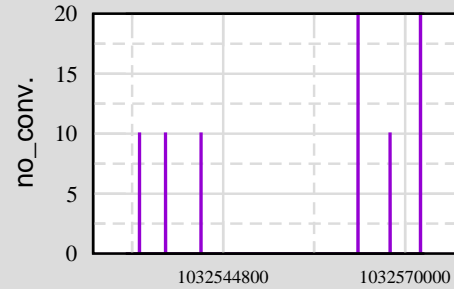
Ch 5: H0:PEM-LVEA_DST9_3
