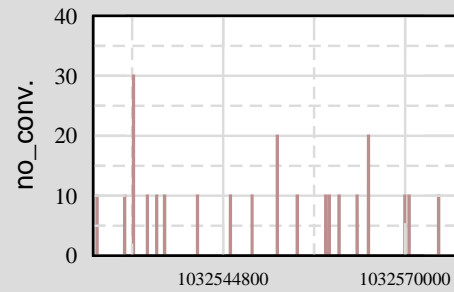
Ch 5: H0:PEM-LVEA_DST9_3
