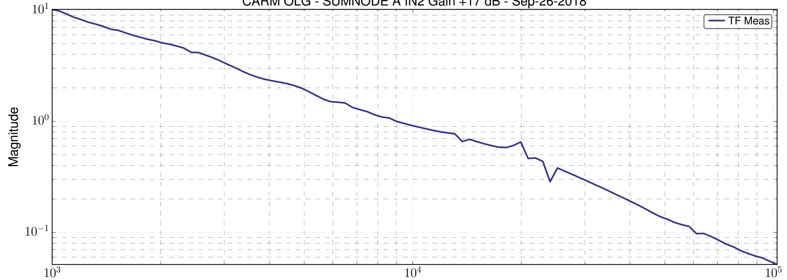
CARM OLG - SUMNODE A IN2 Gain +17 dB - Sep-26-2018
