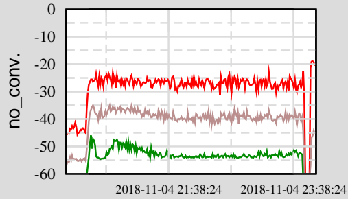
Ch 3: H1:LSC-REFLAIR_A_RF9_DEMOD_RFMON Ch 8: H1:LSC-REFL_A_RF45_DEMOD_RFMON Ch 12: H1:ASC-REFL_A_RF9_DEMOD_RFMON_4 Ch 16: H1:ASC-REFL_B_RF9_DEMOD_RFMON_4
