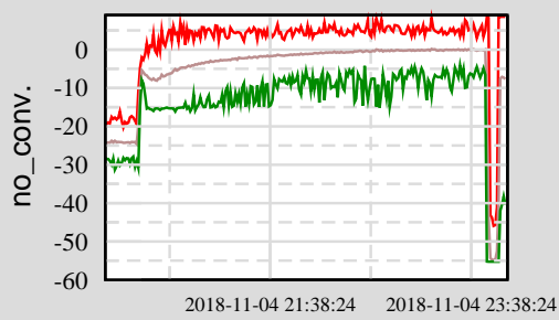
Ch 2: H1:LSC-REFL_A_RF9_DEMOD_RFMON Ch 6: H1:LSC-REFLAIR_B_RF135_DEMOD_RFMON Ch 11: H1:ASC-REFL_A_RF9_DEMOD_RFMON_3 Ch 15: H1:ASC-REFL_B_RF9_DEMOD_RFMON_3
