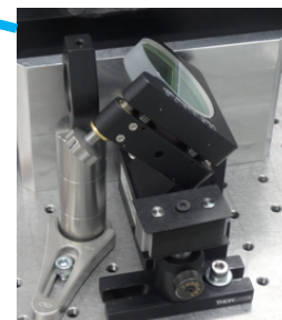
Bottom periscope, IO_MB_M5, 554 Hz
