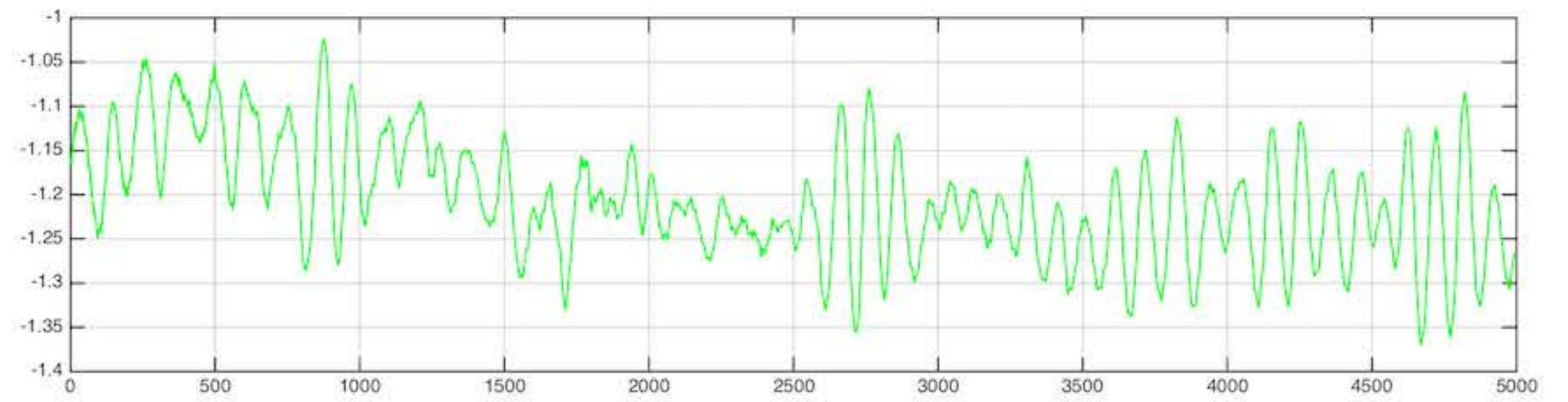
H1:LSC-REFL_A_RF9_I_OUTPUT
