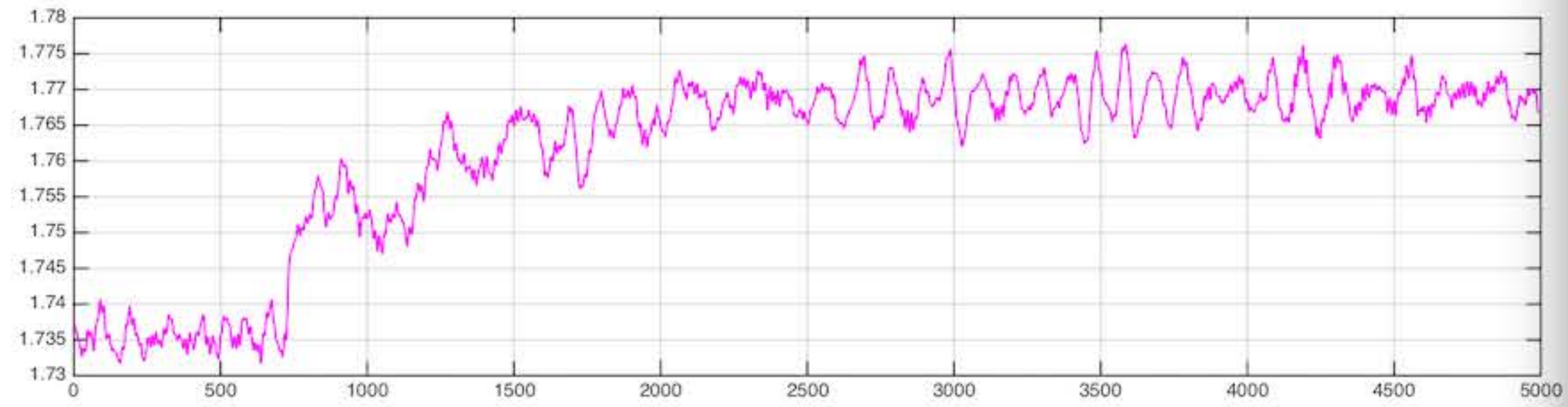
H1:ASC-POP_B_PIT_OUT16
