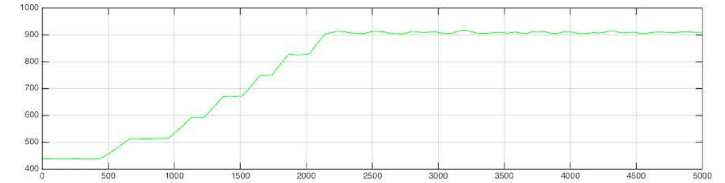
H1:LSC-REFL_A_RF9_I_OUTPUT
