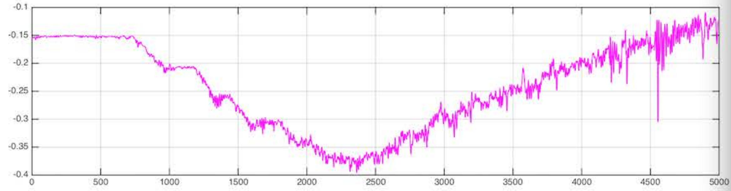
H1:LSC-REFL_B_RF9_Q_OUTPUT
