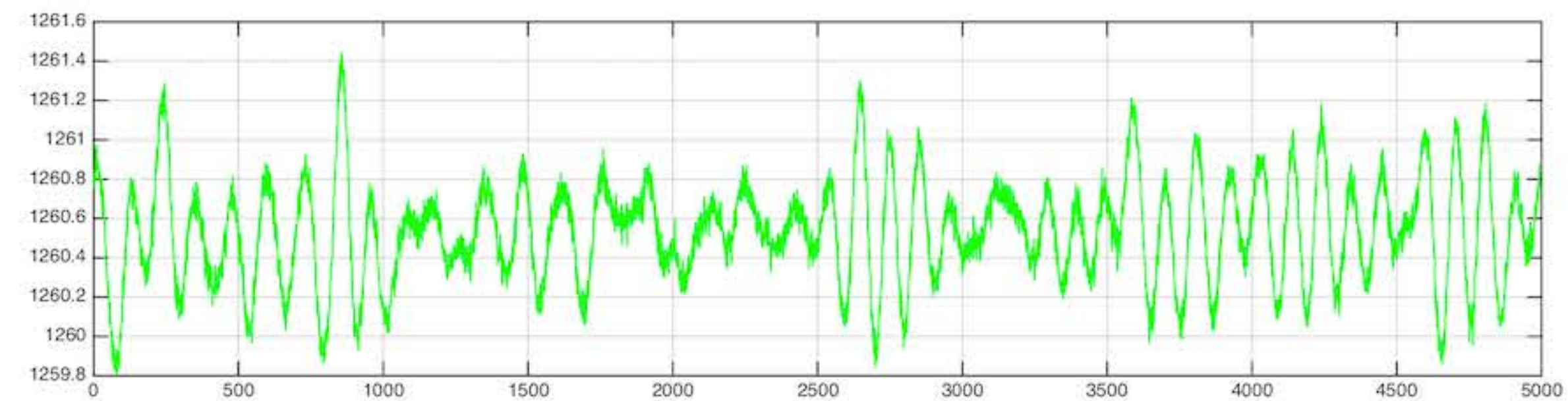
H1:LSC-REFL_A_RF9_I_OUTPUT
