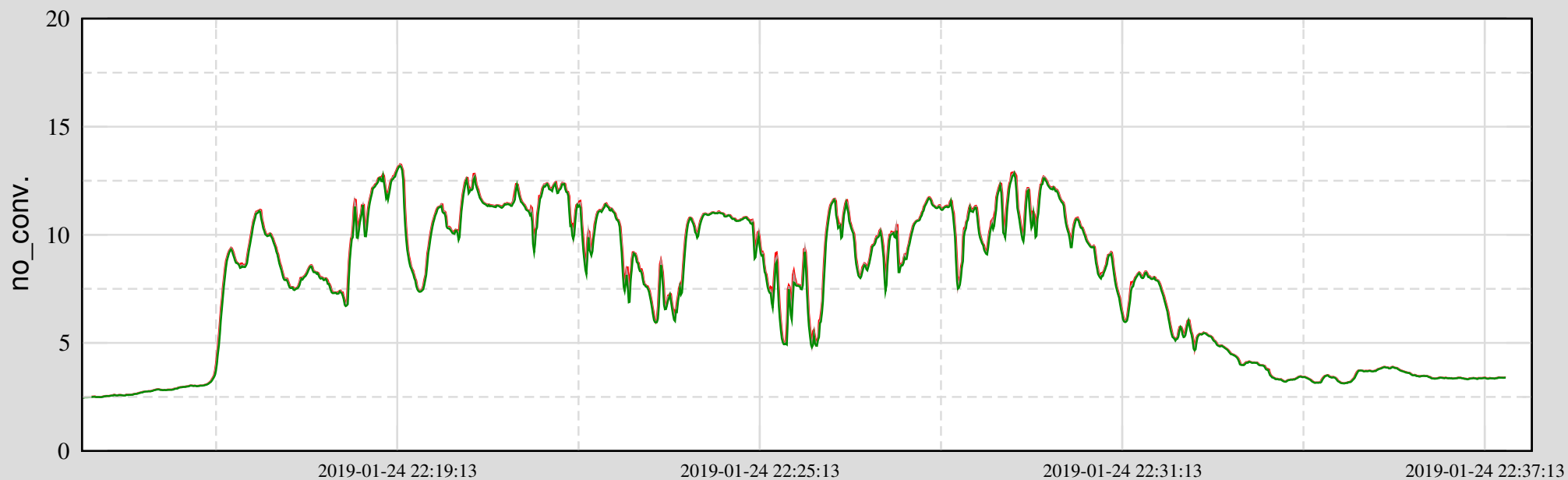
Ch 1: H1:PSL-FSS_PC_MON_OUT_DQ
