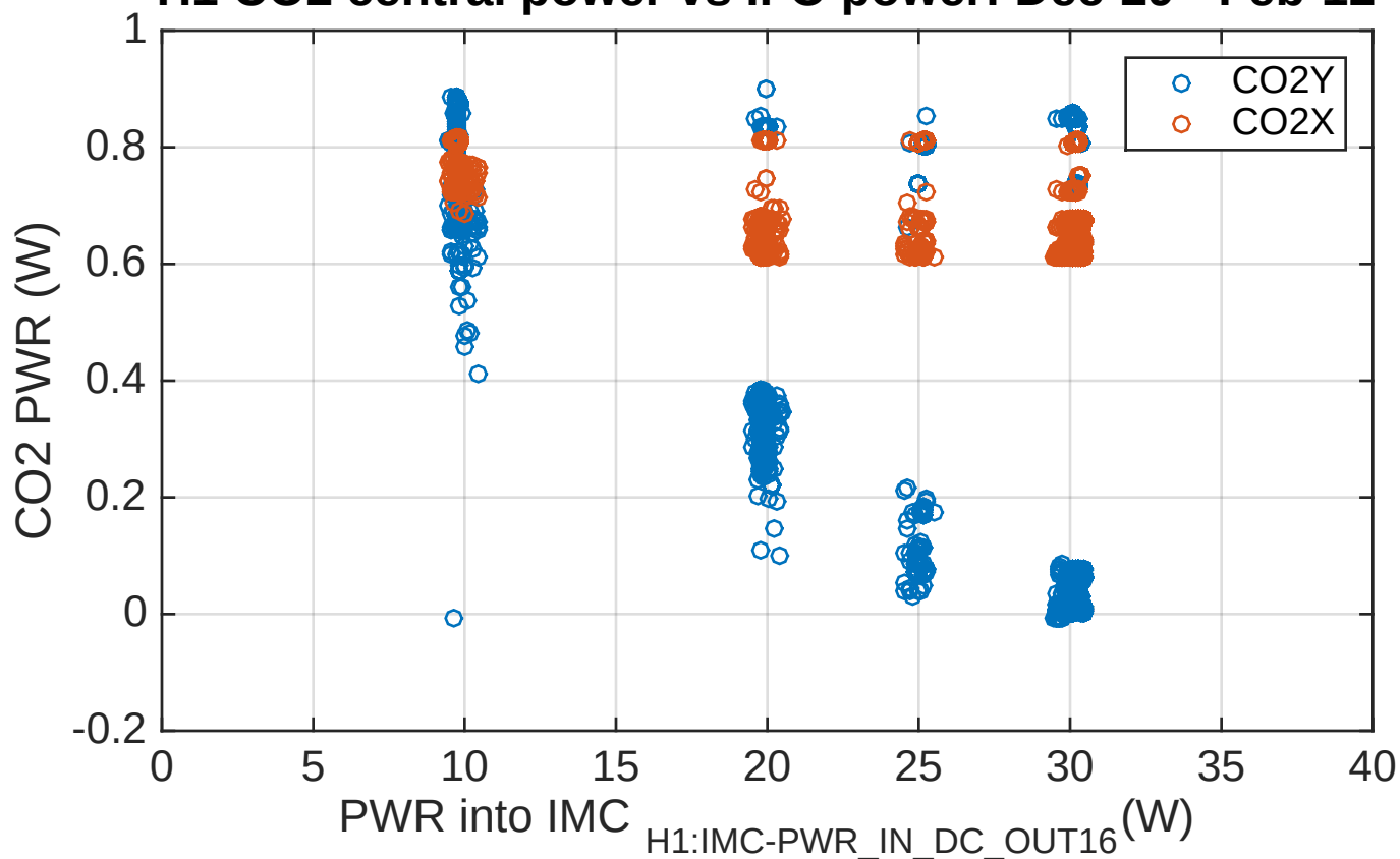
H1 CO2 central power vs IFO power: Dec-29 - Feb-12
