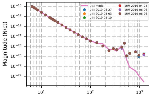
2019-06-26 H1 UIM Actuation Function: (PCAL/iStage SUS EXC) vs. Model
