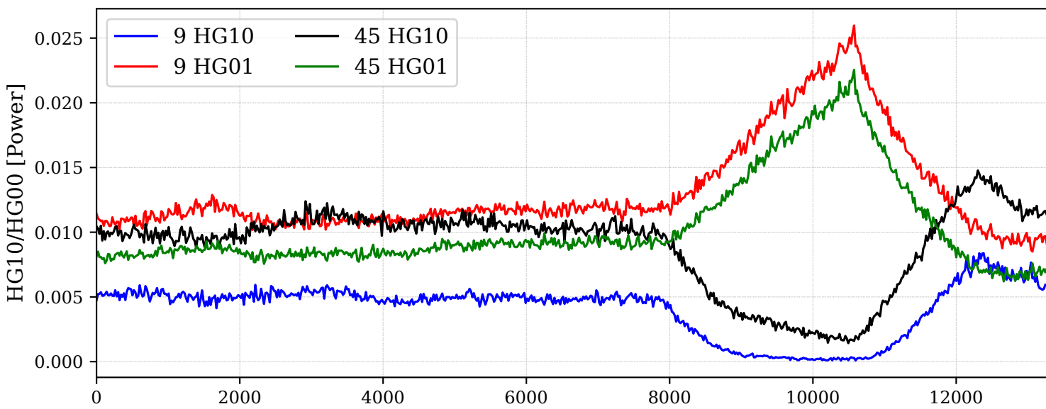
9/45 MHz sidebanda mode content vs CO2
